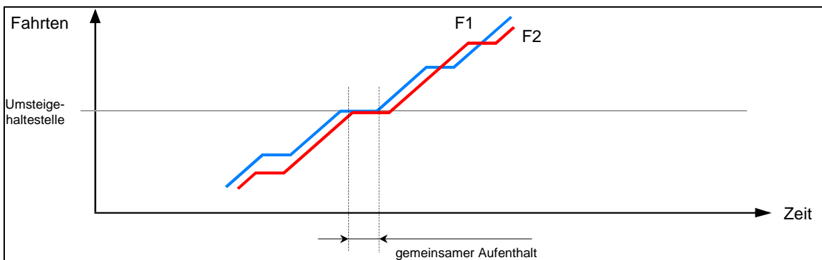
Abb. 3-2: Blockanschluss
