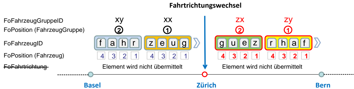
Abbildung 22 Fahrtrichtungswechsel ohne Übertragung "FoFahrtrichtung"
