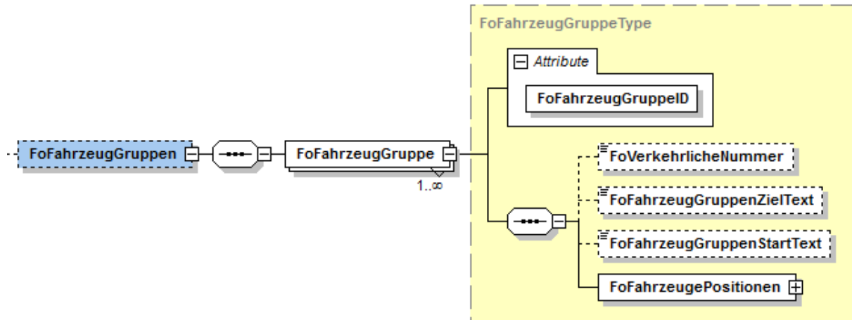
Abbildung 14 Element "FoFahrzeugGruppen"
