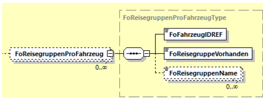
Abbildung 29 Element "FoReisegruppenProFahrzeug"
