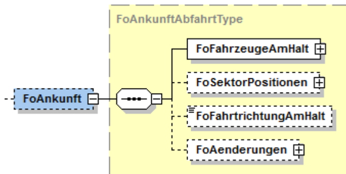
Abbildung 35 Element "FoAnkunft"
