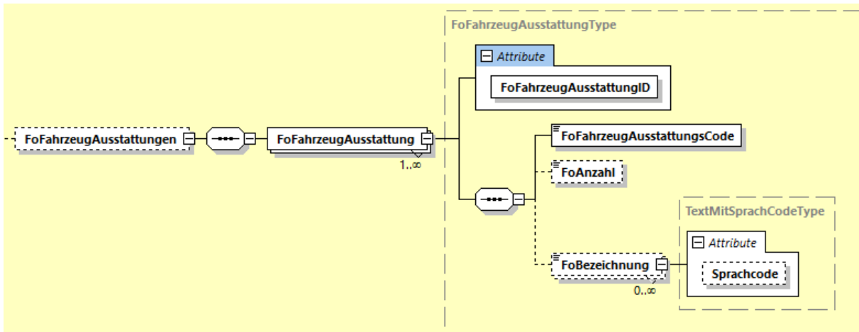
Abbildung 10 Element "FoFahrzeugAusstattungen"
