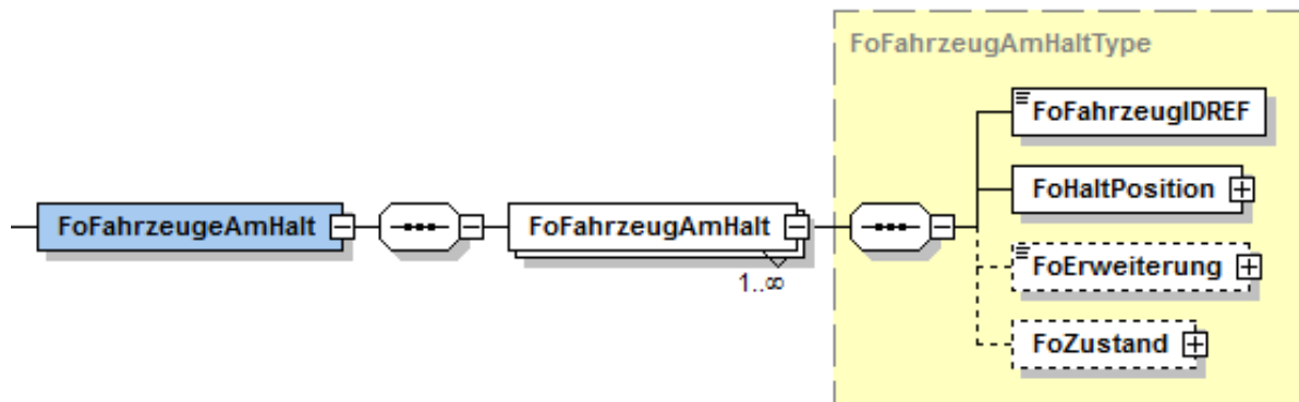
Abbildung 36 Element "FoFahrzeugeAmHalt"
