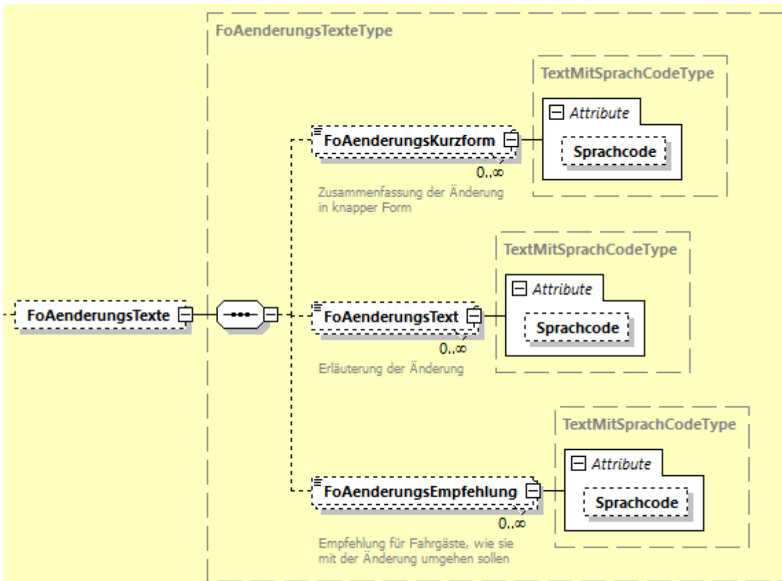
Abbildung 48 "FoAenderungstexte"
