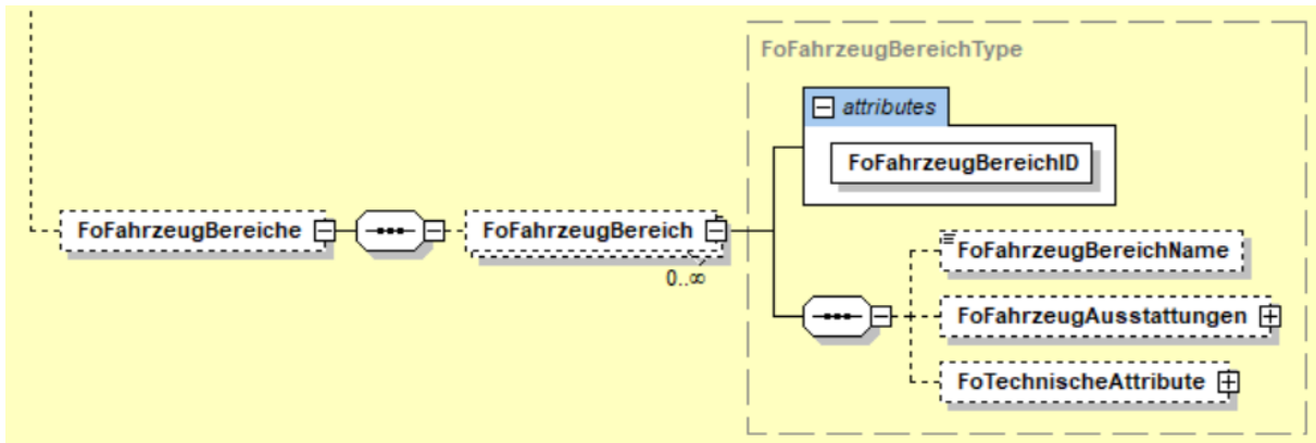
Abbildung 12 – Element "FoFahrzeugBereiche"
