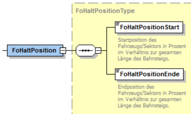
Abbildung 39 Element "FoHaltPosition"
