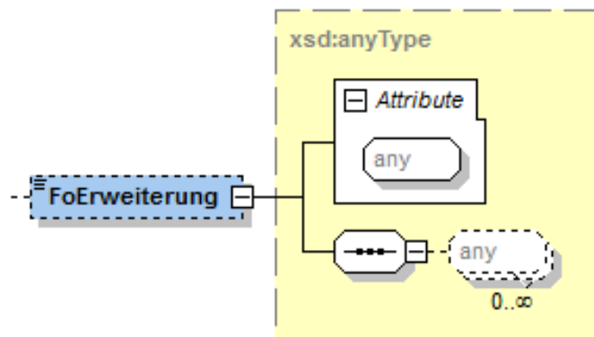
Abbildung 50 Element "FoErweiterung"
