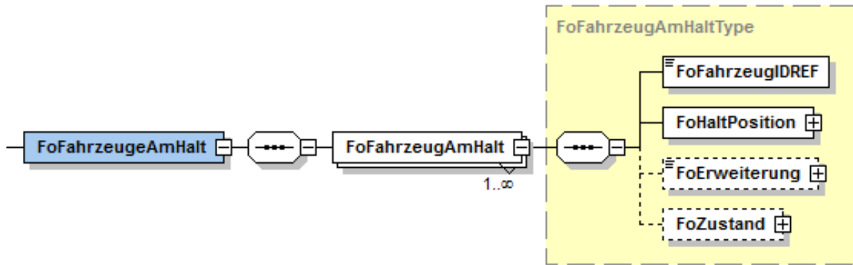
Abbildung 41 Element "FoFahrzeugeAmHalt"
