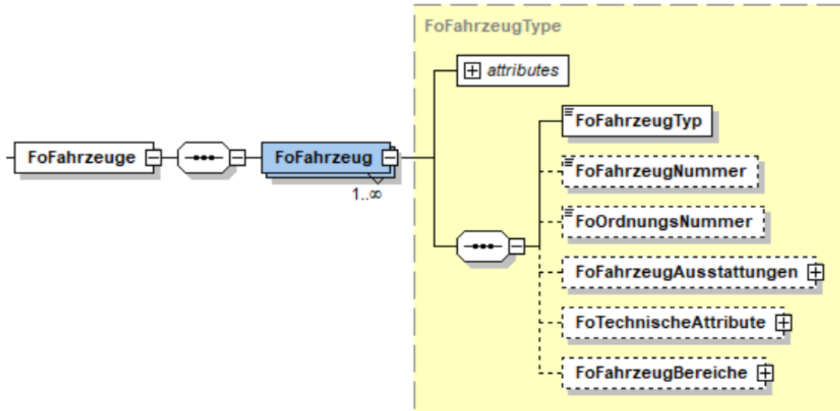
Abbildung 9 Element "FoFahrzeuge"
