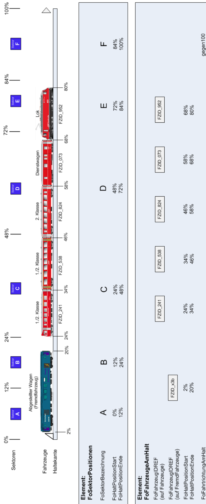
Abbildung 31 HaltPositionen für Fahrzeuge und Sektoren an der Haltekante
