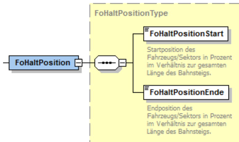
Abbildung 37 Element "FoHaltPosition"
