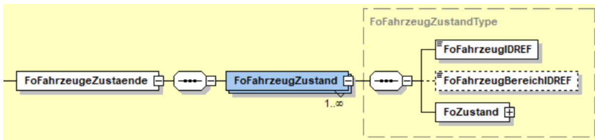
Abbildung 27 Element "FoFahrzeugeZustaende"
