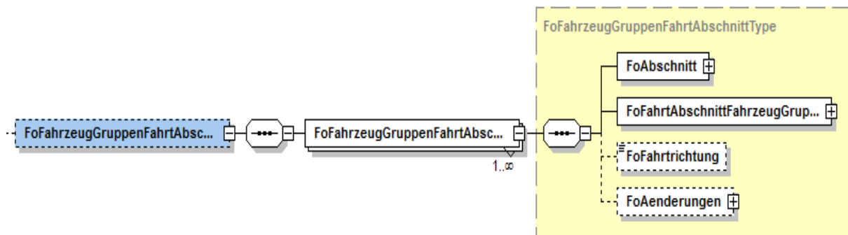
Abbildung 17 Element "FoFahrzeugGruppenFahrtAbschnitte"
