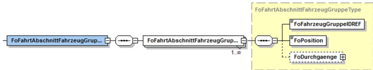
Abbildung 19 Element "FoFahrAbschnittFahrzeugGruppen"
