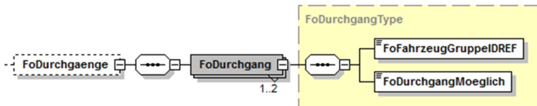
Abbildung 20 Element "FoDurchgaenge"
