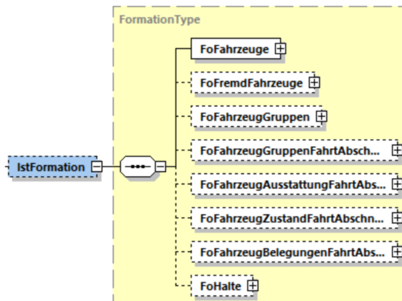
Abbildung 8 Element "IstFormation"
