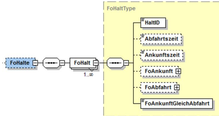
Abbildung 30 Element "FoHalte"
